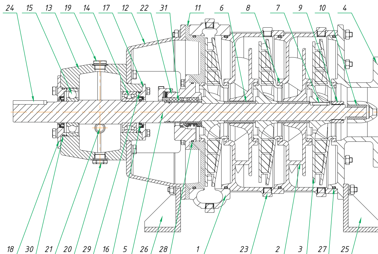
Центробежный насос НЦ.3-127P1.Riflon (6"x5"x14"). Конструкция.
